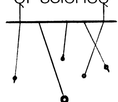
PENDULUM
